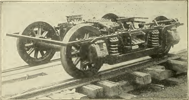
Fig. 13. Heavy M. C. B. Truck
